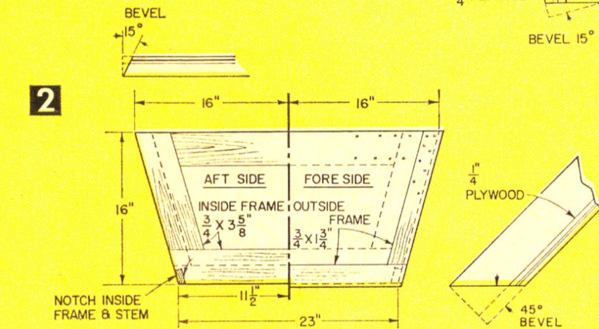
C STEM & FRAME
